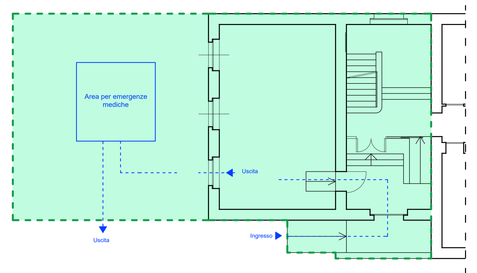
Planimetria generale dell'area per l'accettazione, da utilizzare in caso di maltempo - Scala 1:100
