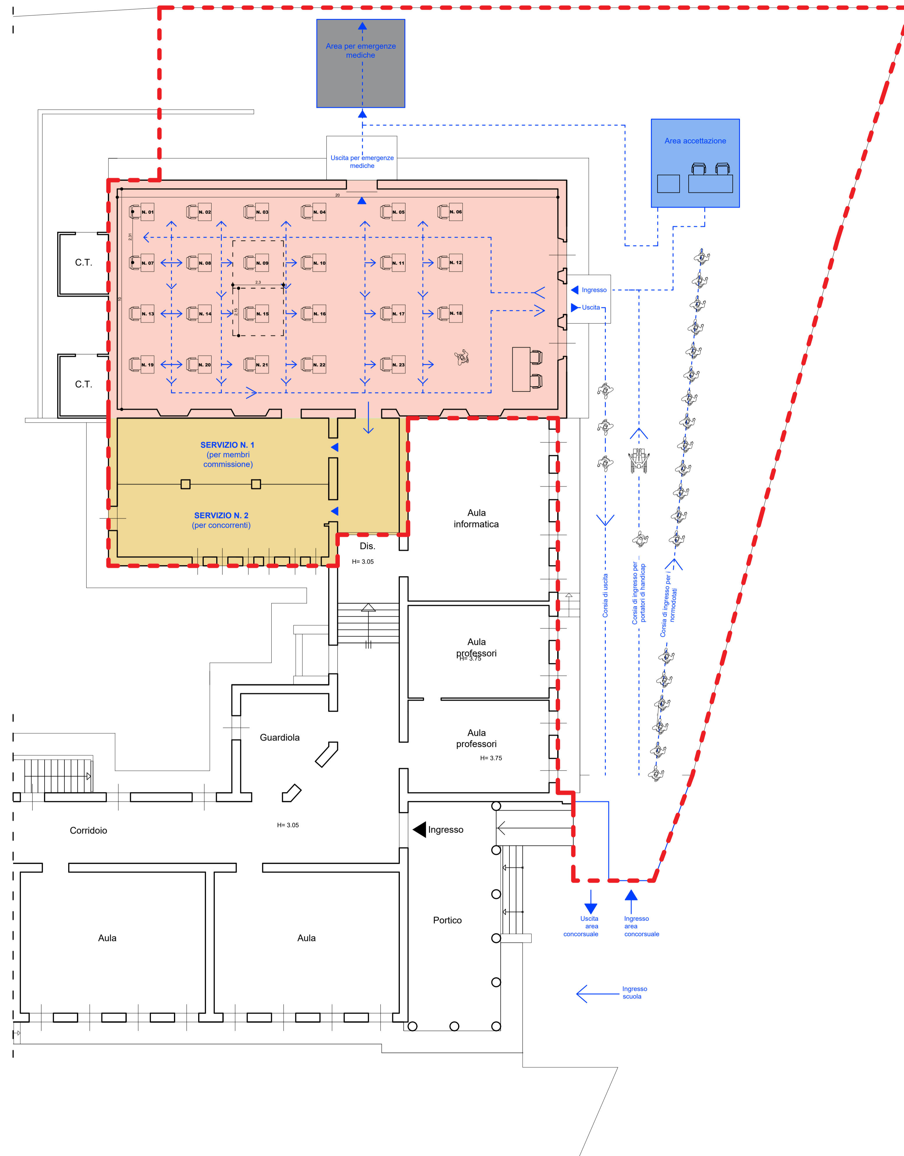
Planimetria generale delle aree per lo svolgimento del concorso - Scala 1:100
